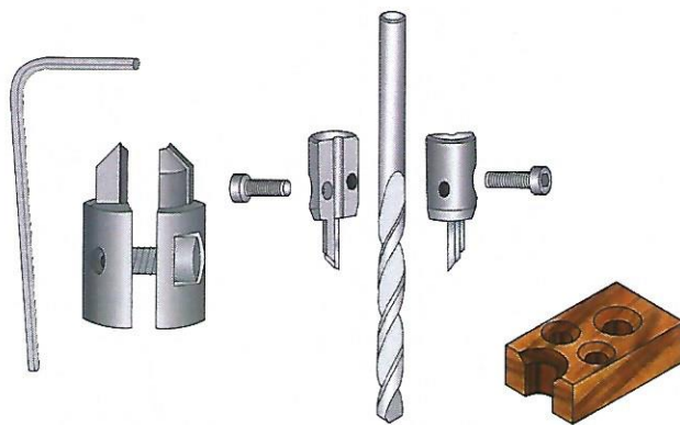
Escareador Regulável
