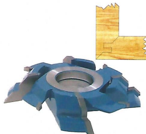
Fresa Widia Rejunte em Meia Esquadria
